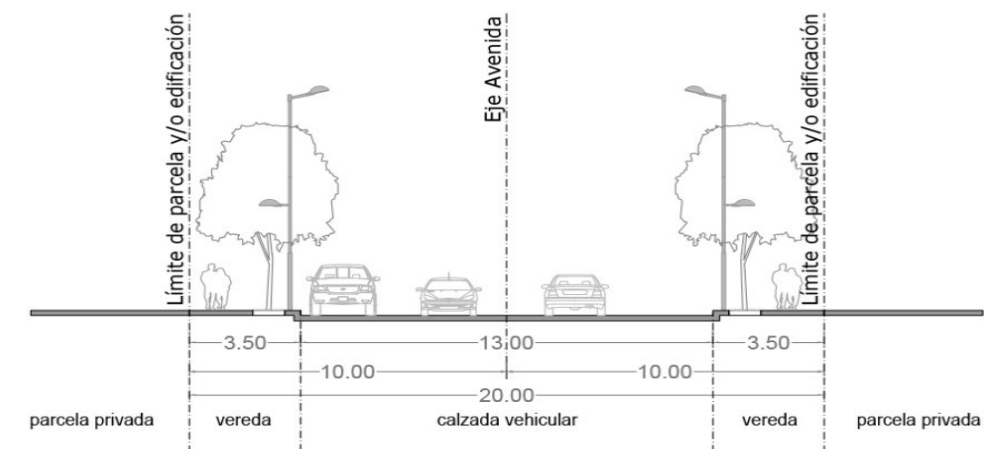
Fig. 9: Sección transversal de Vías Avenidas Tipo 6.
