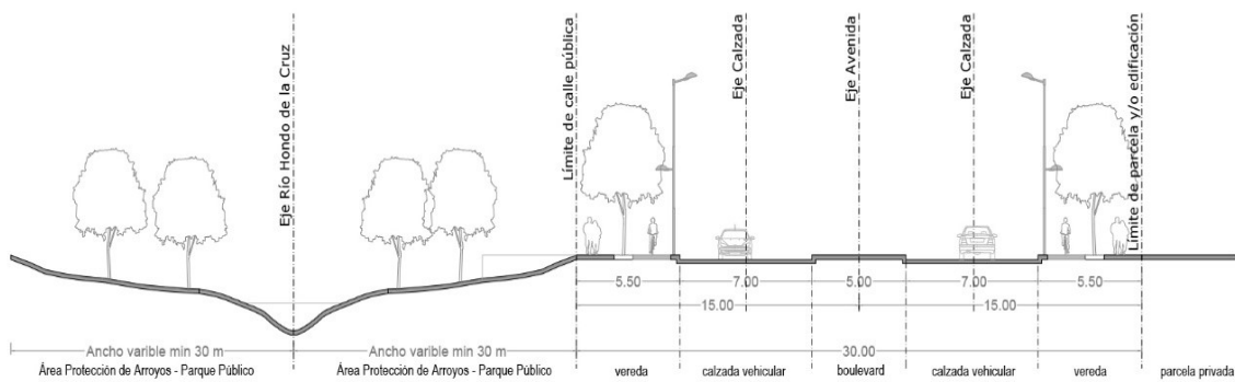
15: Sección transversal de Vías Especiales Tipo 2.
