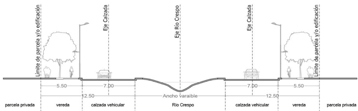
Fig. 17: Sección transversal de Vías Especiales Tipo 4. MODIFICAR ANCHO DE CALLE A 15 CON VEREDA CONTIGUA A ARROYO CRESPO (MODIFICAR NOMBRE: ES ARROYO CRESPO)
