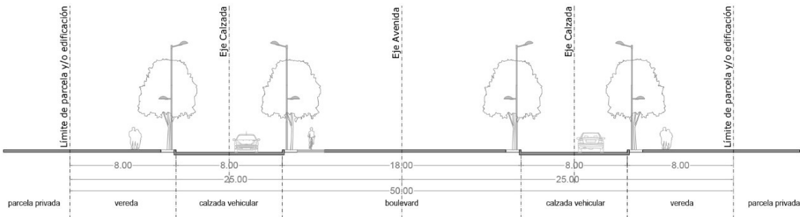
Fig. 4: Sección transversal de Vías Avenidas Tipo 1.
