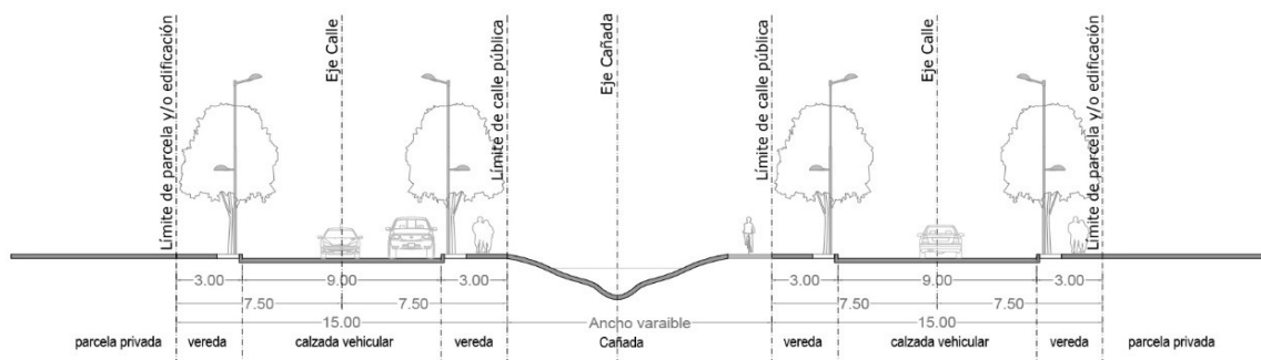
Fig. 16: Sección transversal de Vías Especiales Tipo 3. ACOTAR ANCHO DE BICISENDA (2 M)
