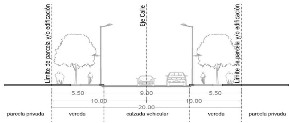
Fig. 11: Sección transversal de Vías Calles Tipo 8.
