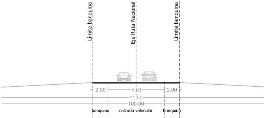
Fig. 3: Detalle Calzada vehicular de la Ruta Nacional.
