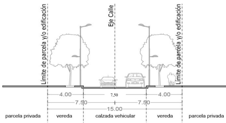
Fig. 13: Sección transversal de Vías Calles Tipo 10. Calzada de 7,50
