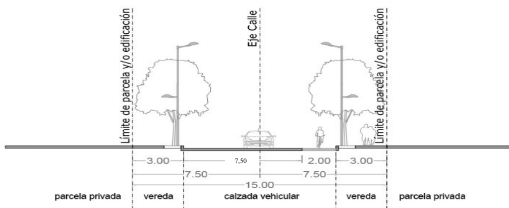
Fig. 18: Sección transversal de Vías Especiales Tipo 4. Calzada de 7,50
